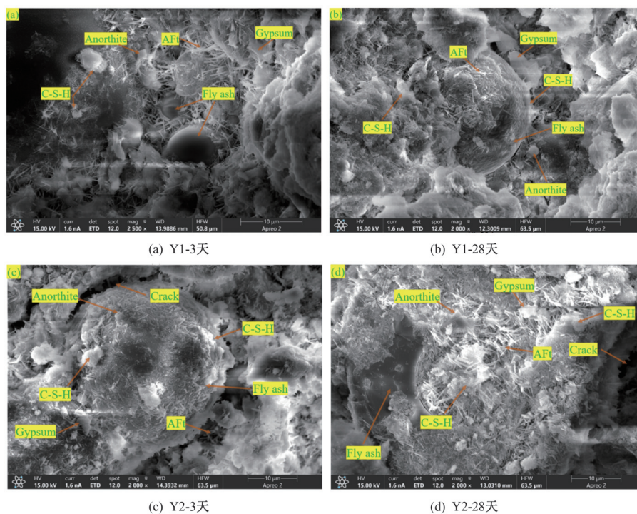
图 8 固废基胶凝材料 3 天、28 天龄期的 SEM 图
