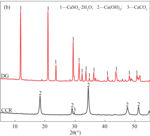
(b) 固废激发剂 图 2 原材料 XRD 图谱 Fig. 2 XRD pattern of raw materials
